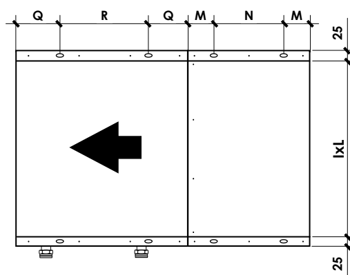
Dimensioni Generali unità – Unit general dimensions
