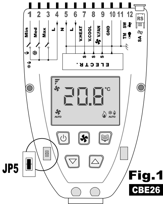
Schema elettrico interno Internal wiring diagram
